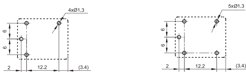
安装孔尺寸 (底视图)
