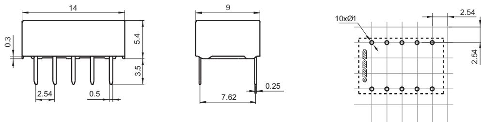
安装孔尺寸 (底视图)
