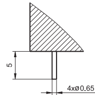
引出端形式 1 (焊针式)
